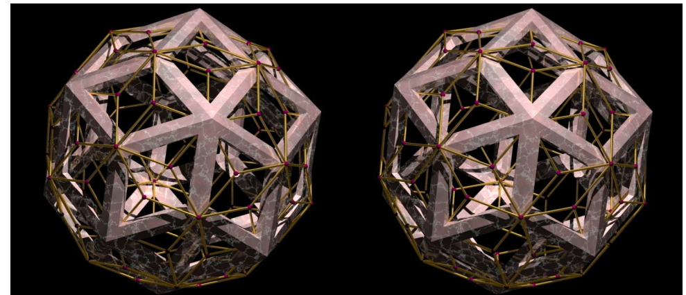
Triacontaèdre enchaîné par Ennéacontaèdre - Image : Edmond Bonan
