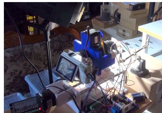
Rail de stacking. 11 pièces imprimées, 2 moteurs pas à pas et un contrôleur Arduino.
