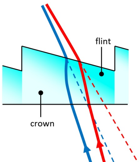
Fig. 5 : Prisme des lunettes Chromadepth Les zones les plus compressées ont un indice plus élevé et plus dispersif (flint), que les autres (crown), ce qui permet de restituer les zones rouges en avant de l'image réelle.
