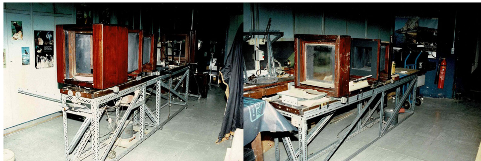
Appareil OP3000 transformé en banc de reproduction macro, reportage Alain Bonnet
