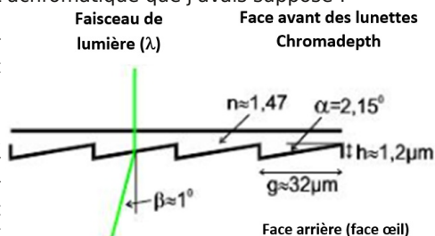
Coupe transversale d'un réseau Chromadepth.
