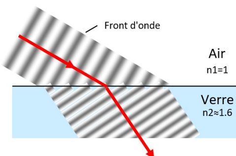
Fig. 1b - Réfraction : représentation ondulatoire.
