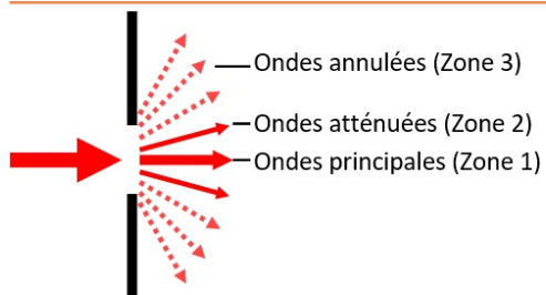
Fig. 2a - Diffraction par une pupille. Représentation par des flèches indiquant les sens de propagation.
