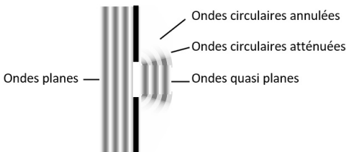
Fig. 2b - Diffraction par une pupille. Représentation ondulatoire simplifiée.
